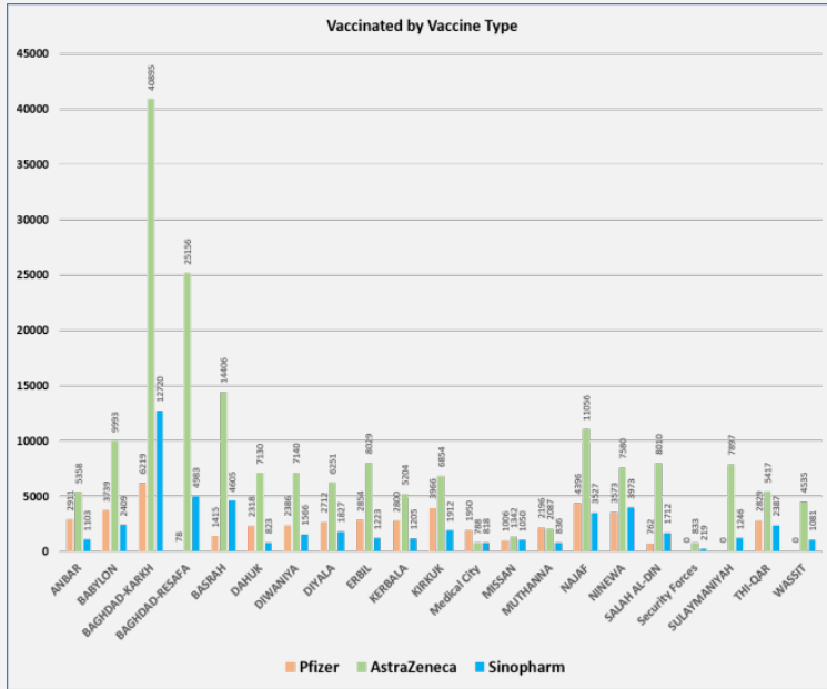
الشكل 8: التطعيم حسب أنواع اللقاحات المستخدمة
