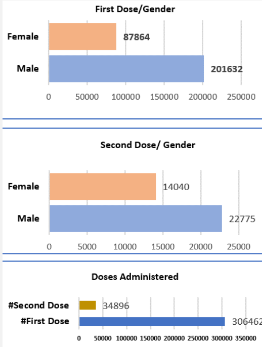
الشكل 7: حالة التطعيم بحسب الجرعات
