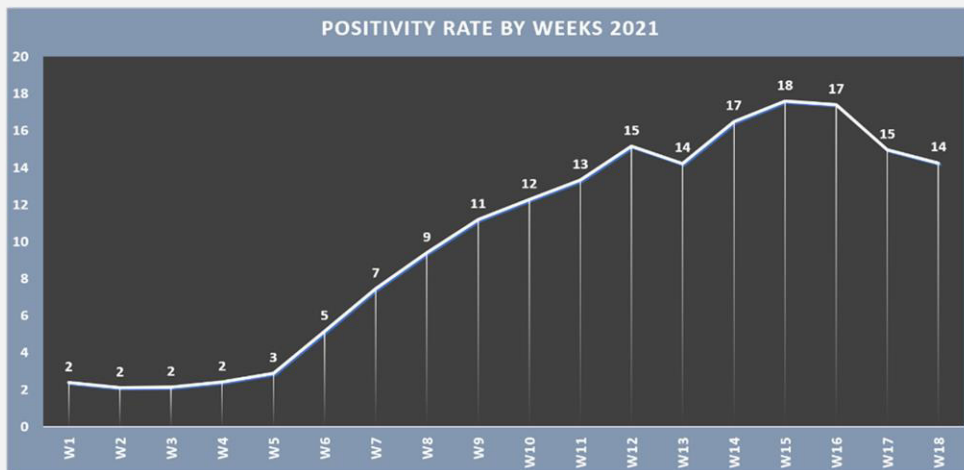
الشكل 4: معدل الإيجابية حسب الأسابيع 2021
