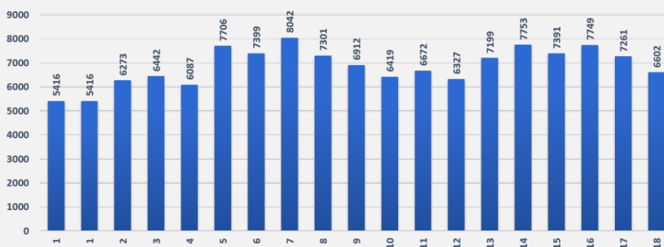
الشكل 2: عدد الفحوصات لكل مليون
