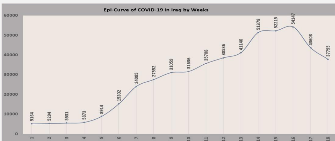
الشكل 1: المنحنى الوبائي للمرض في العراق للأسبوع 18
