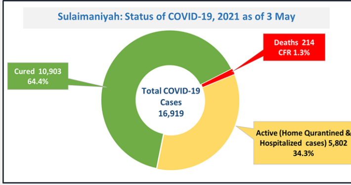
الشكل 9: حالة كوفيد-19 في محافظة السليمانية، حتى 3 مايو/أيار 2021
