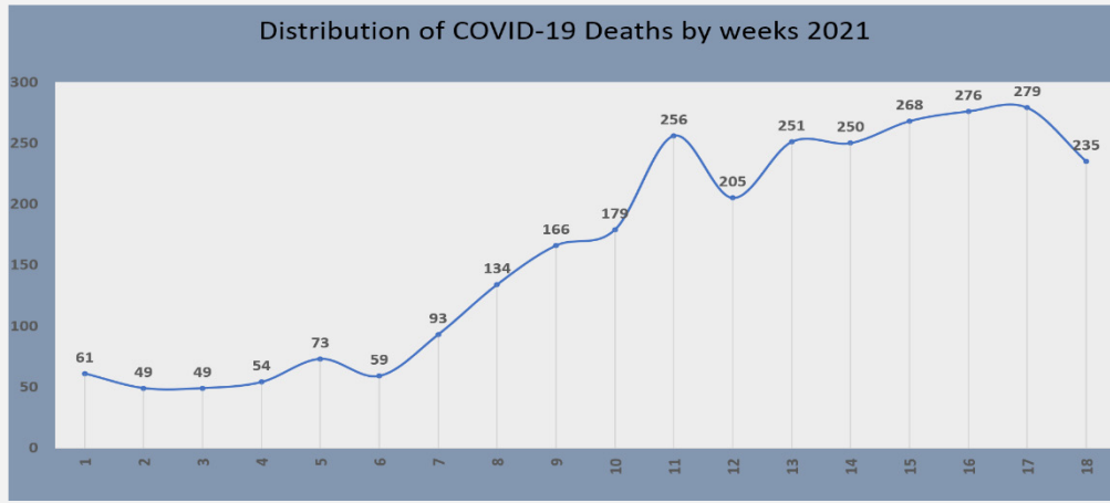
الشكل 5: توزيع وفيات كوفيد-19 في أسابيع 2021
