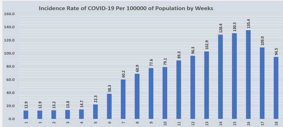
الشكل 3: معدل الإصابات بكوفيد-19 لكل 100,000 من السكان أسبوعياً
